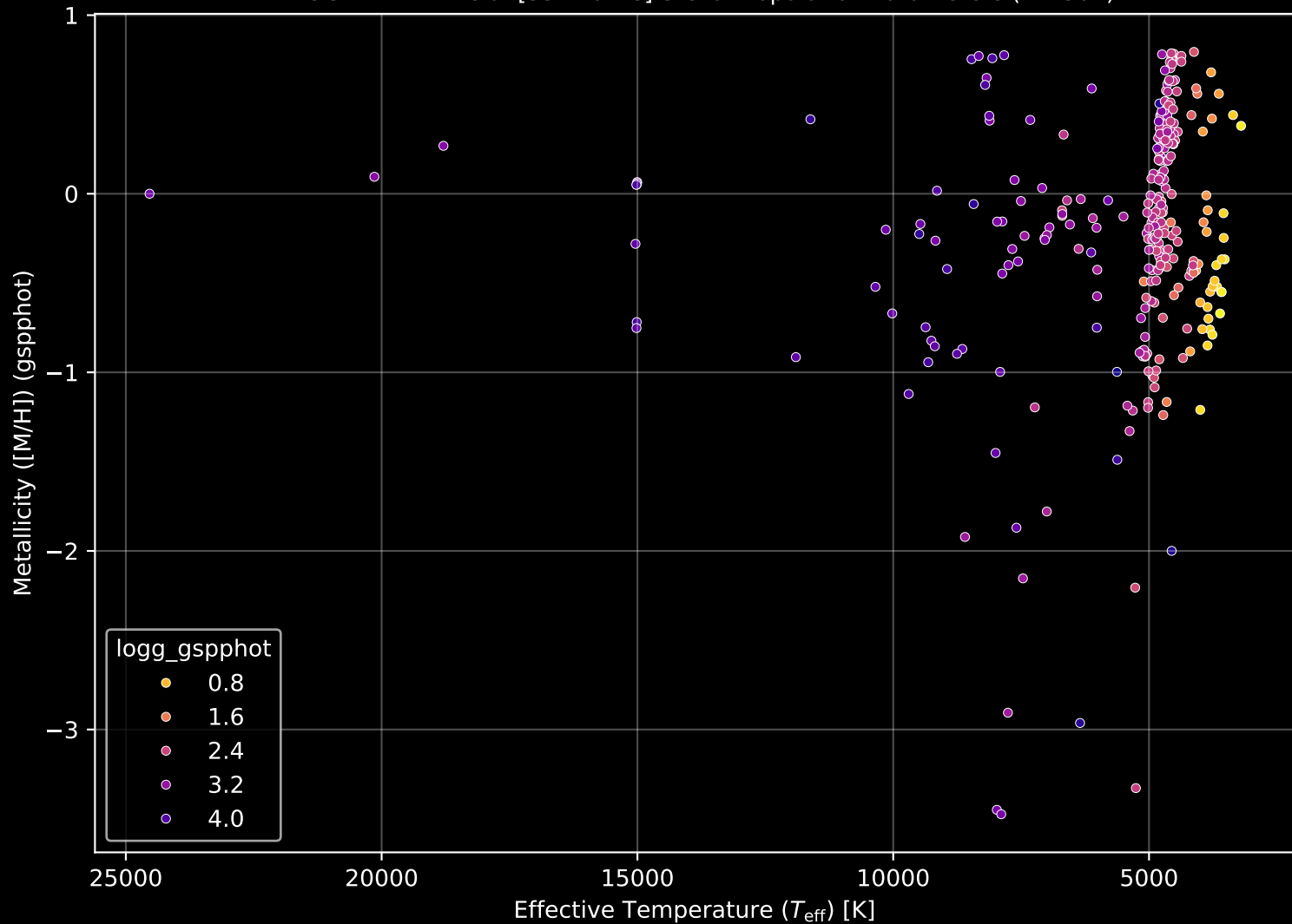
APOGEE DR17 Field: [357+02-C] Stellar Population Parameters (n= 302)
